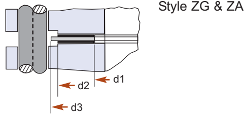
Style ZG & ZA
